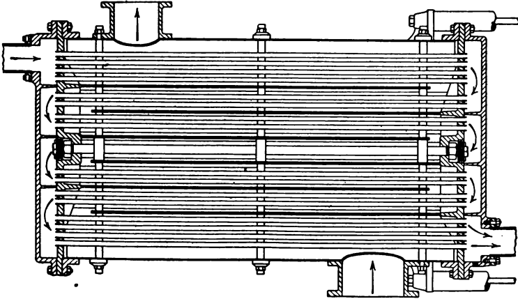
FIG. 59.—Nordberg intercooler.
